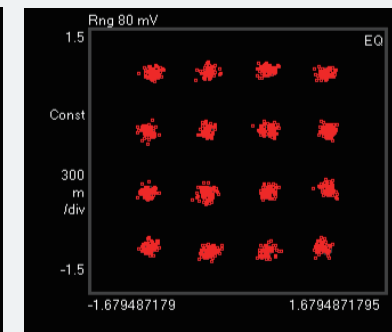
光回路による事前補償時の16QAM信号
