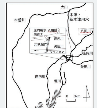
全体図: 国土地理院地図に筆者加筆改訂 部分略図: 資料と現地調査より筆者作成 Fig.1 木曾川からの幹線水路と河川的位置関係 [「農業水利施設を介した堀川の水質改善に関する試案と課題」(杉浦・田島, 2024) (2024年12月掲載予定)より引用]
