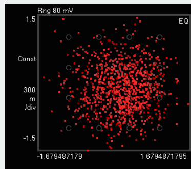
通常の光ファイバ伝送の16QAM信号
