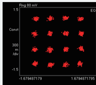
光回路による事前補償時の16QAM信号
